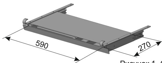
Рисунок 1- Основные размеры
